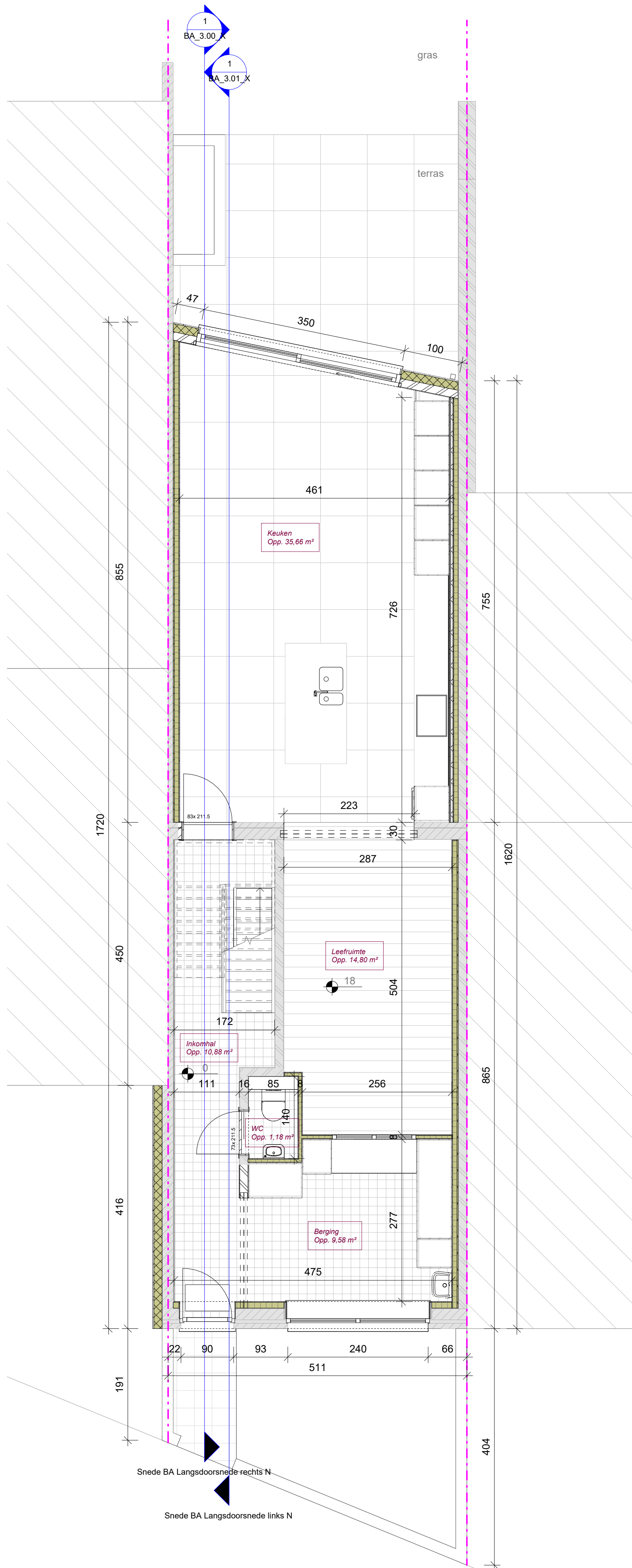
BA_1.00_X P_N_1.00_Grondplan Gelijkvloers
