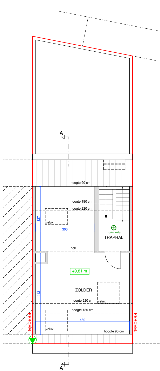
ZOLDER bestaande toestand
