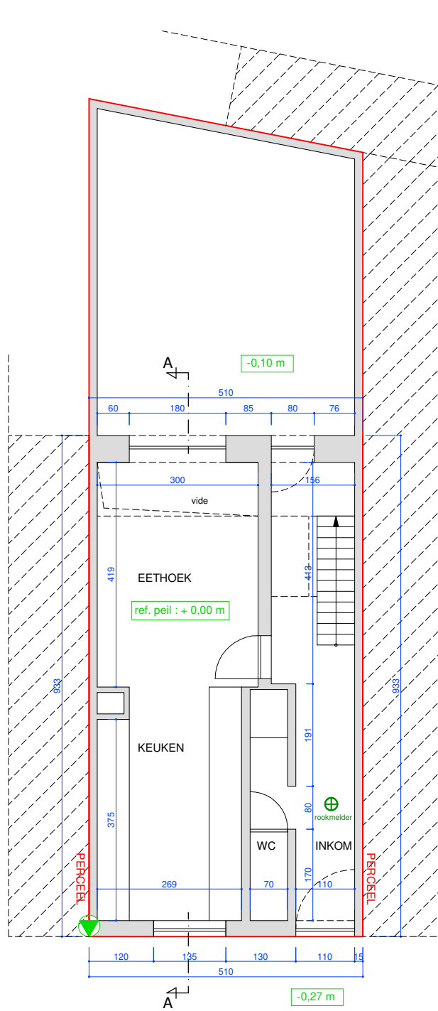
GRONDPLAN bestaande toestand ongewijzigd
