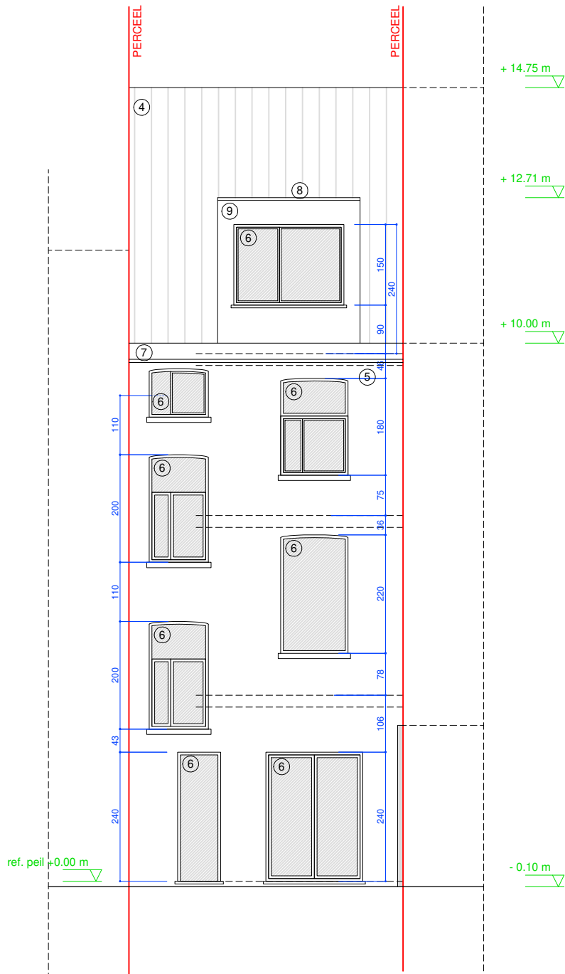
ACHTERGEVEL nieuwe toestand
