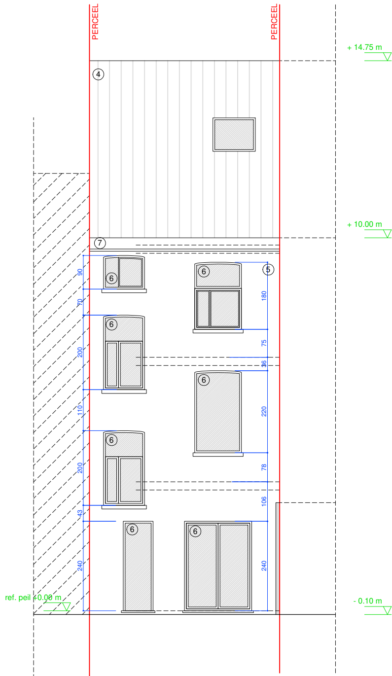
ACHTERGEVEL bestaande toestand
