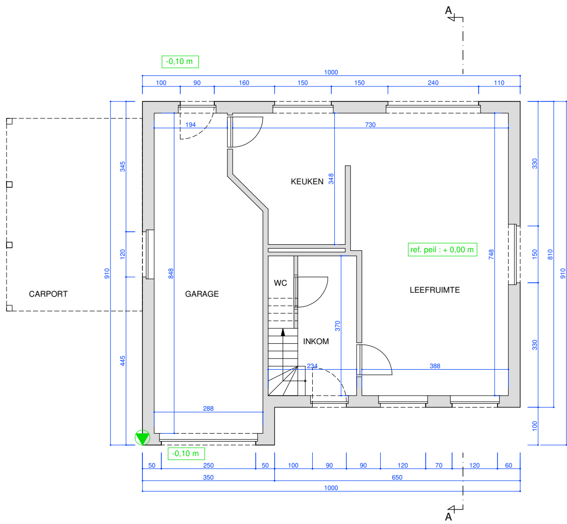
GRONDPLAN bestaande toestand
