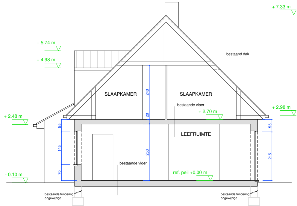
SNEDE AA bestaande toestand
