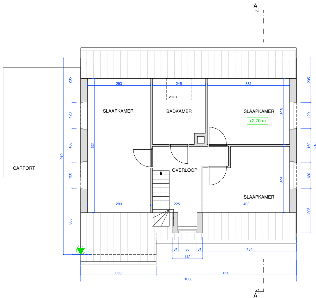
VERDIEPING 1 bestaande toestand
