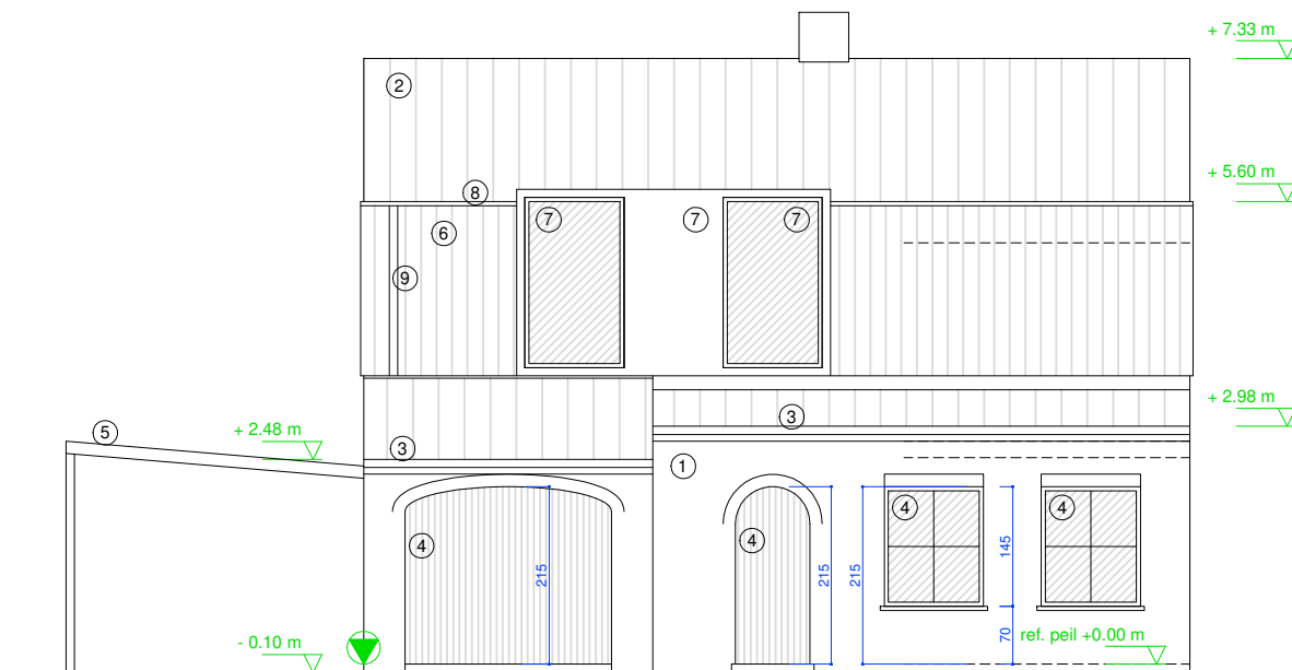
VOORGEVEL nieuwe toestand
