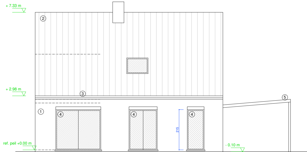
ACHTERGEVEL bestaande toestand
