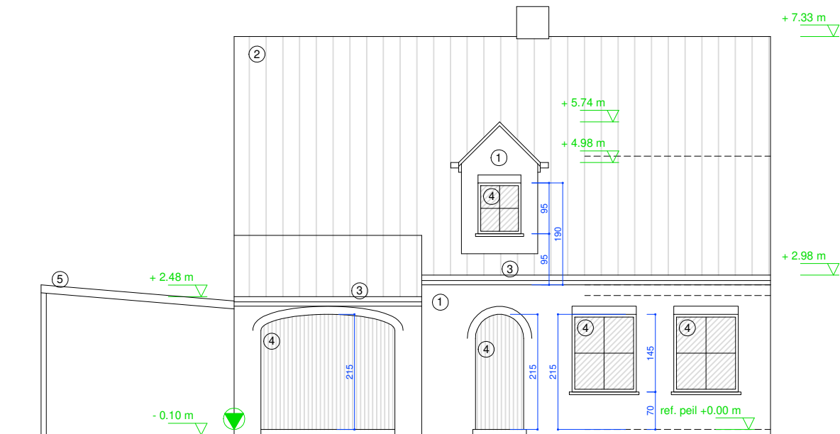
VOORGEVEL bestaande toestand
