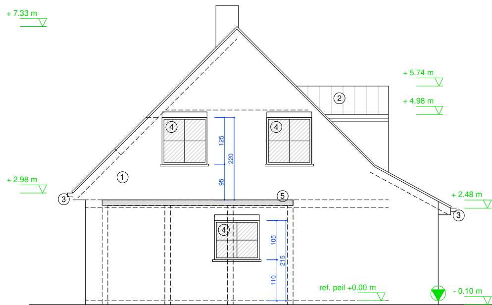
ZIJGEVEL LINKS bestaande toestand
