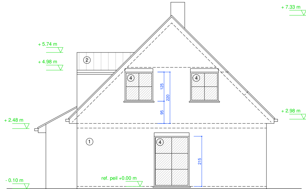
ZIJGEVEL RECHTS bestaande toestand
