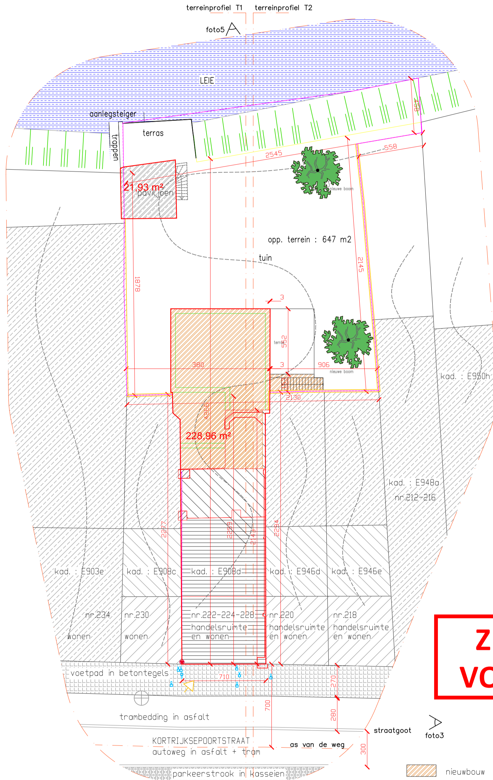
NIEUWE TOESTAND - INPLANTINGSPLAN schaal 1/200 - A3
