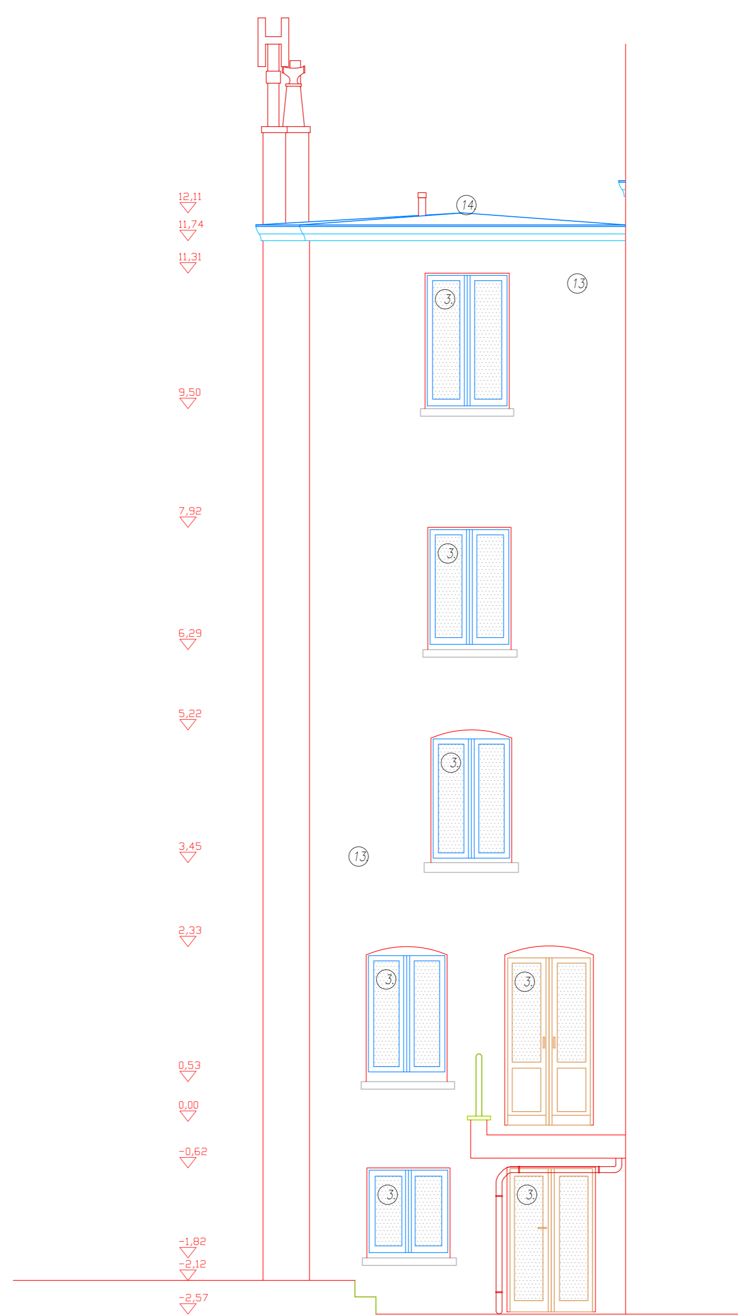
BESTAANDE TOESTAND - LINKERGEVEL schaal 1/50 - A2
