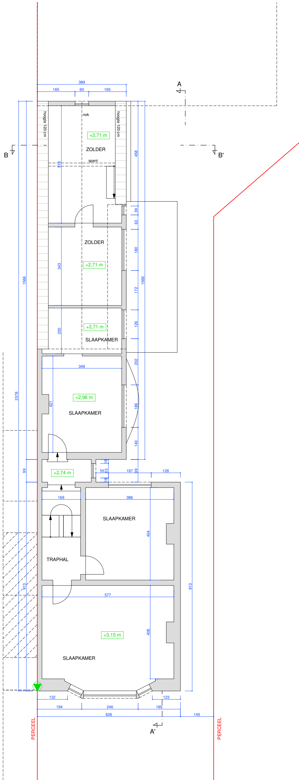
VERDIEPING 01 bestaande toestand
