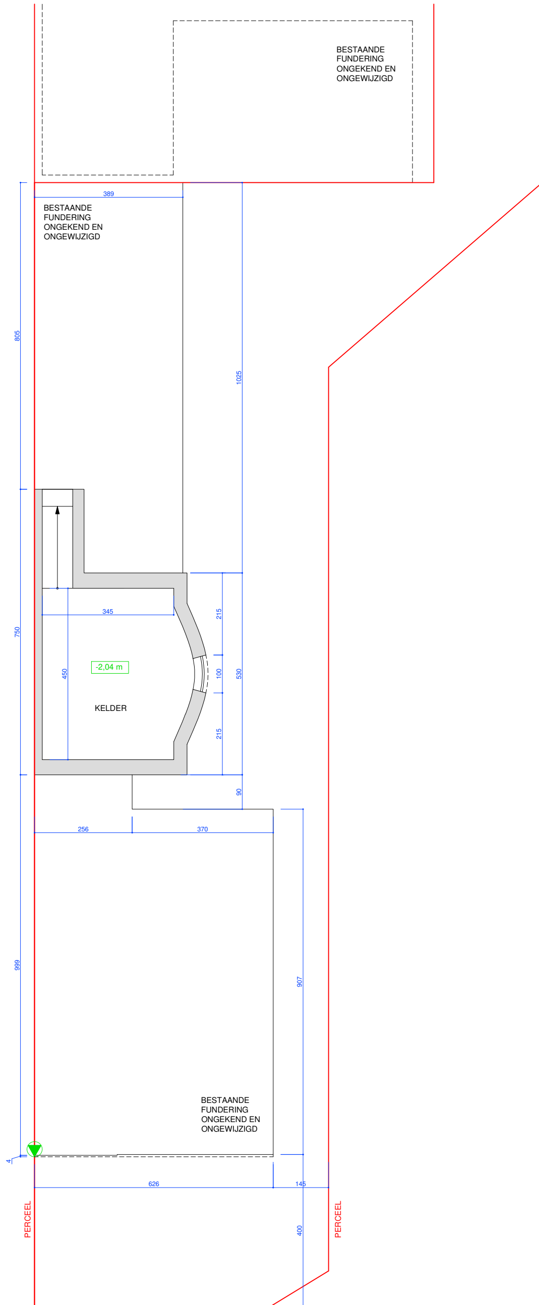
FUNDERINGS -EN RIOLERINGSPLAN bestaande toestand
