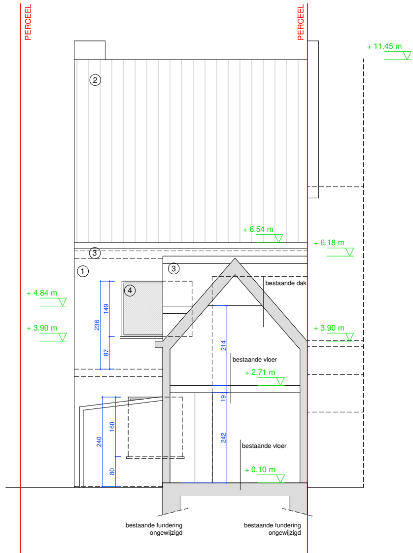
ACHTERGEVEL & SNEDE BB bestaande toestand
