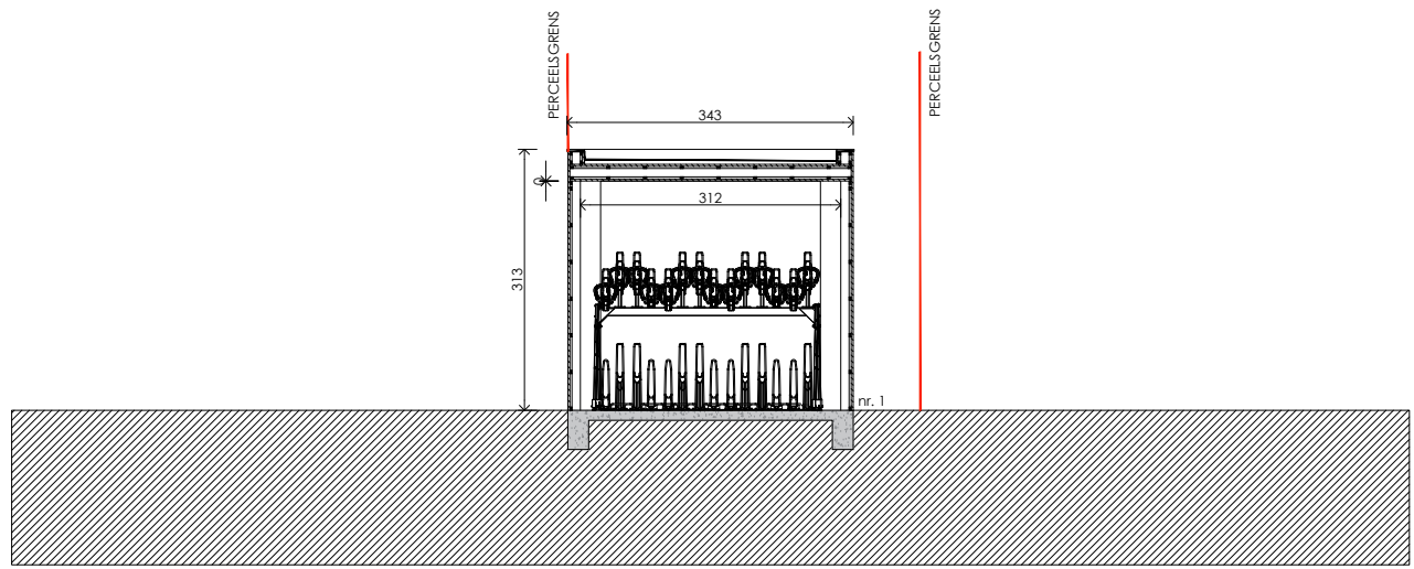
Snede AA'
