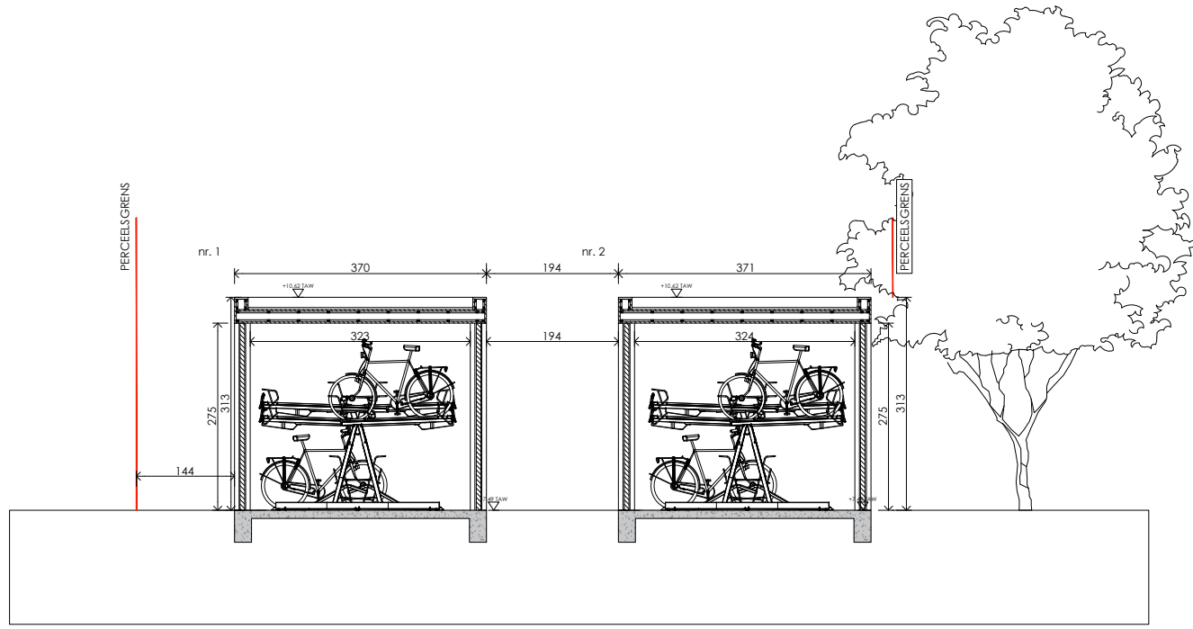
Snede BB'
