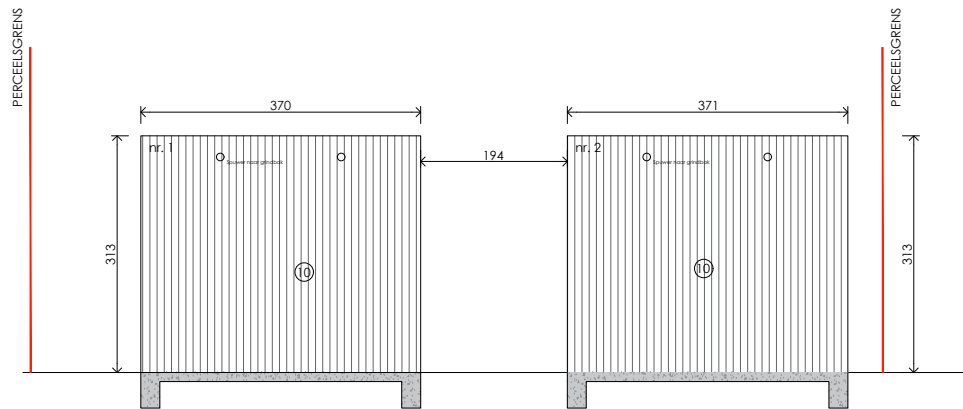
Voorgevel
