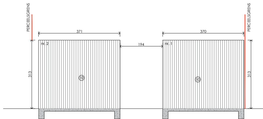
Achtergevel
