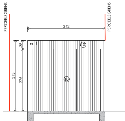
Rechter zijgevel
