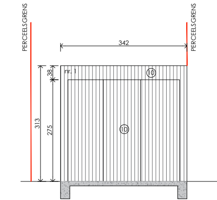
Rechter zijgevel
