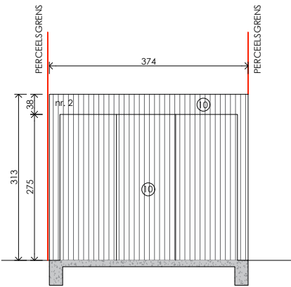
Rechter zijgevel
