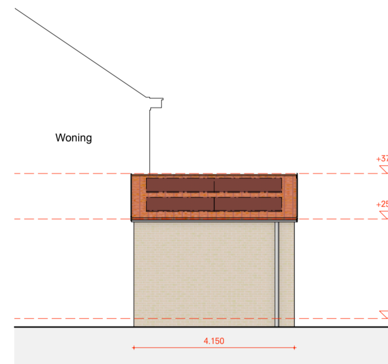
Achtergevel TJF-1
