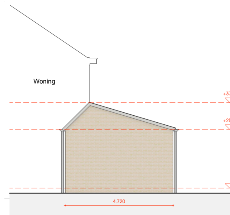
Rechterkopgevel
