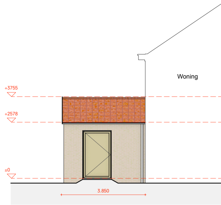
Voorgevel TJF-1
