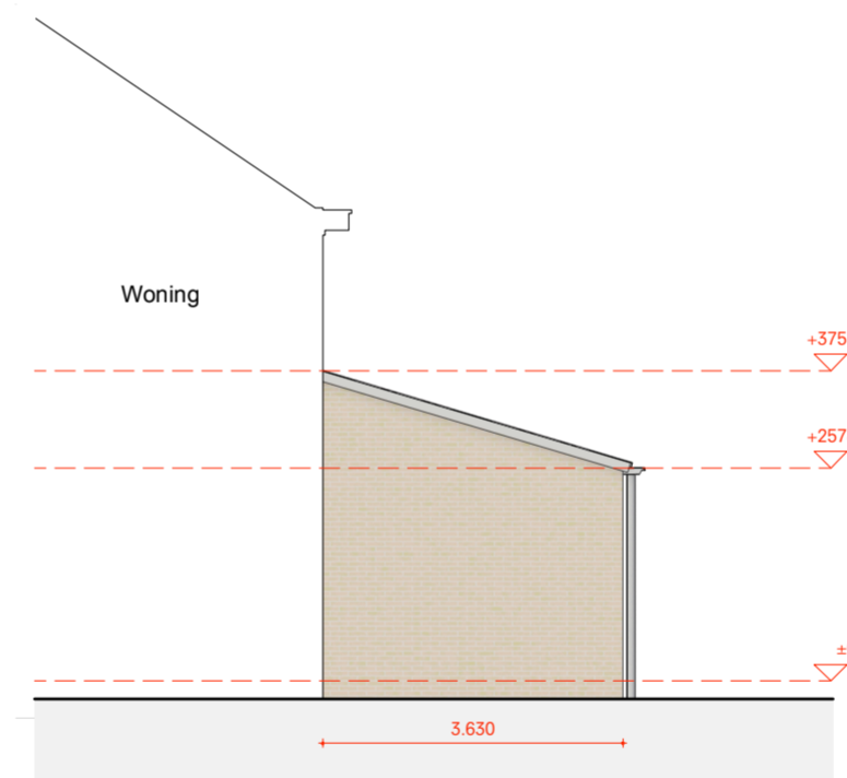
Rechterkopgevel
