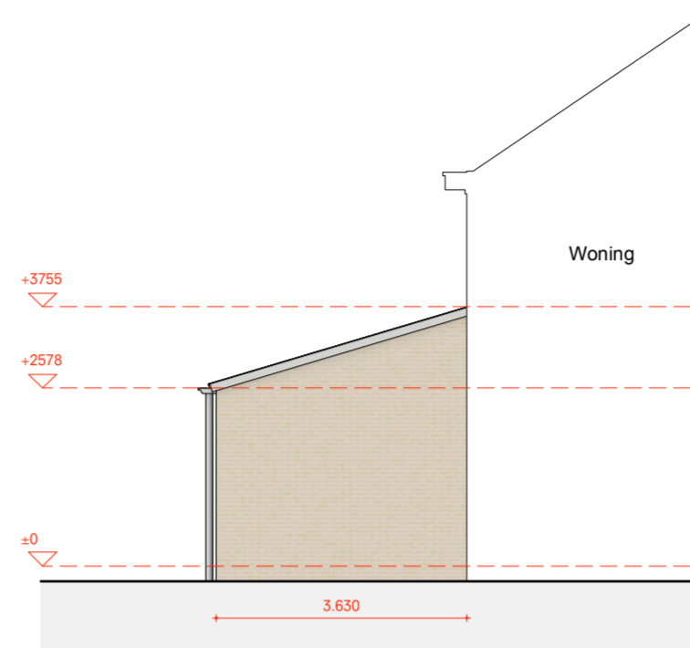
Linkerkopgevel
