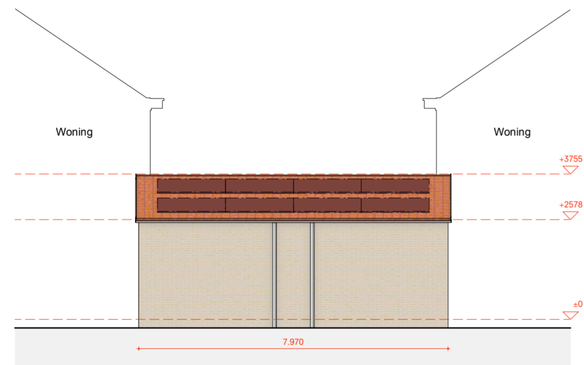
Achtergevel
