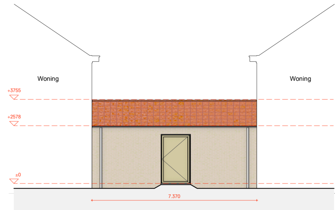
Voorgevel
