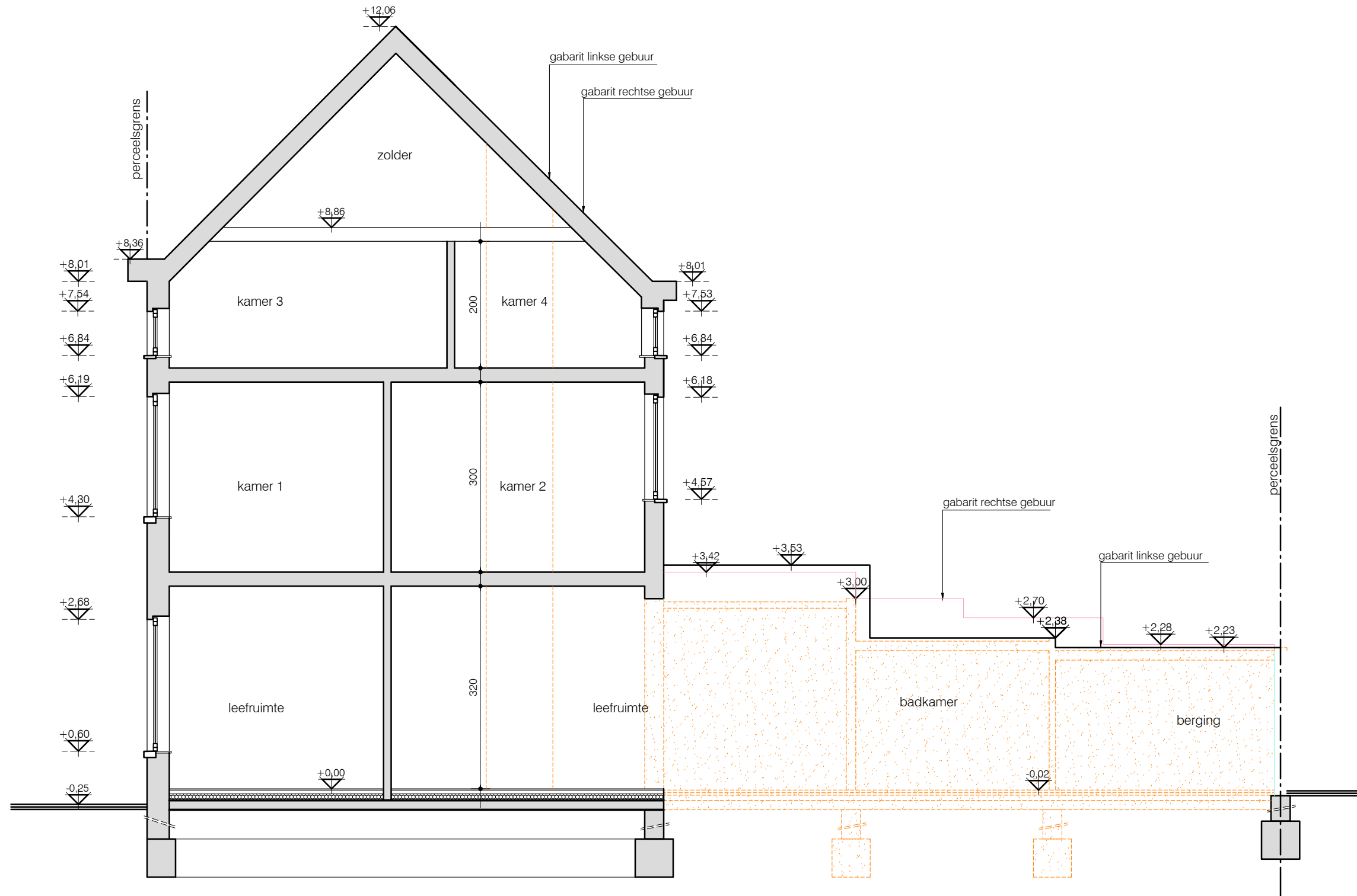
DOORSNEDE A-A Bestaande toestand alle afmetingen zijn in cm
