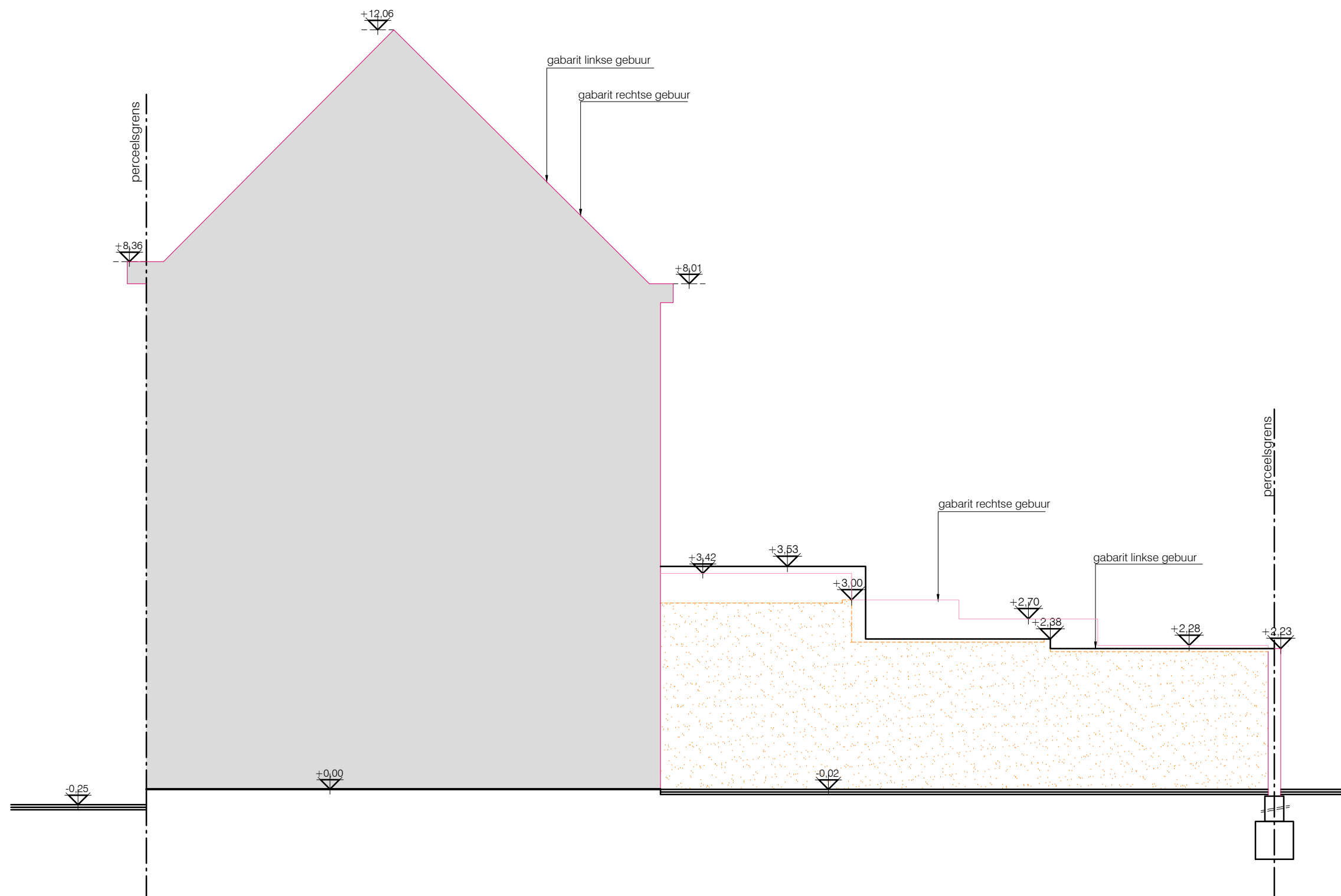
TERREINPROFIEL Bestaande toestand alle afmetingen zijn in cm
