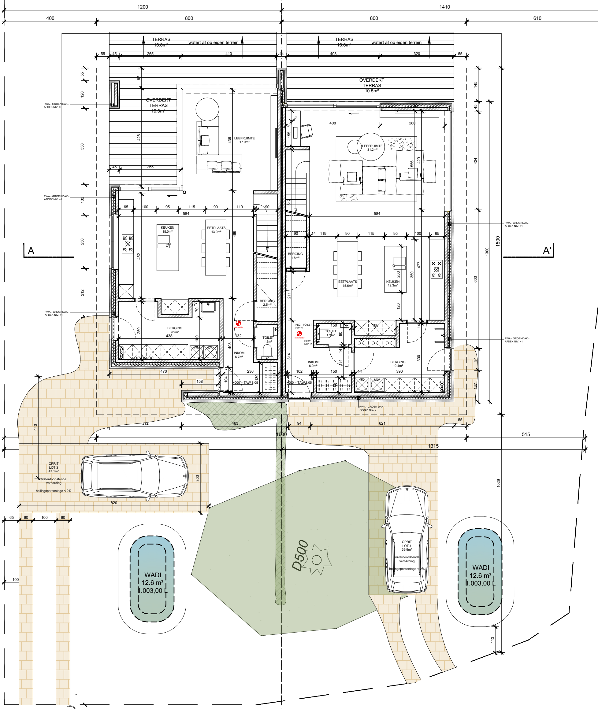
PLAN NIVEAU 0 - LOT 3 WONING - BRUTO OPP. : 84.1m 2 (excl. luifels en tuinmuren)
