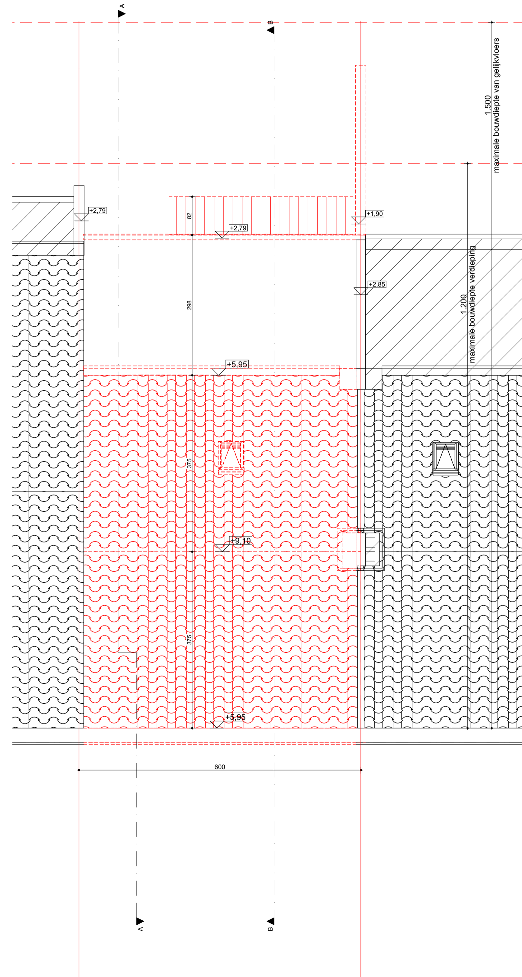
B_P Dak 1:50
