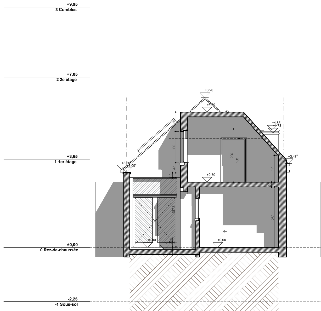
doorsnede BB - vergund Scheldestraat 72, 9040 Gent
