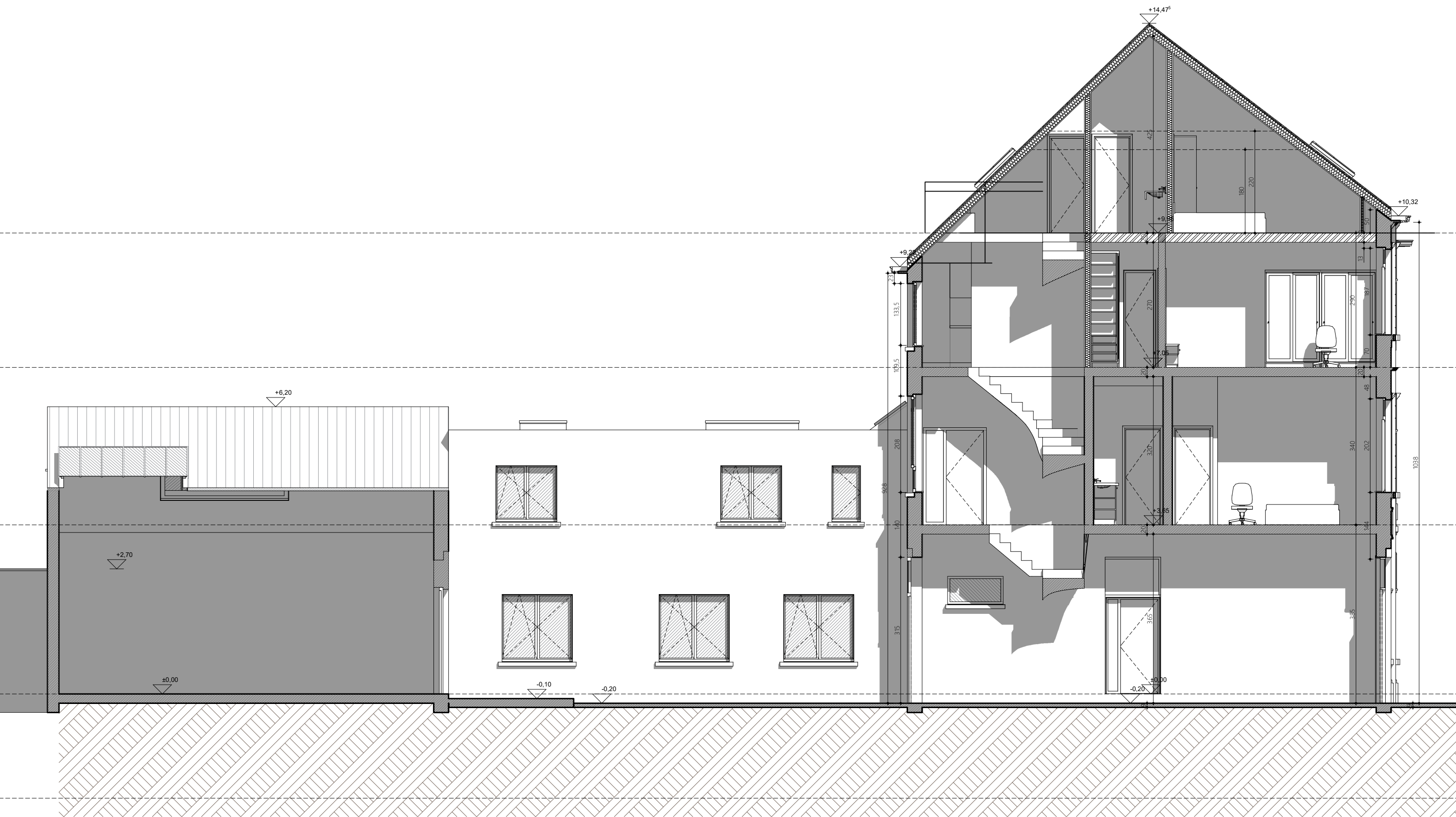
doorsnede AA - huidig Scheldestraat 72, 9040 Gent
