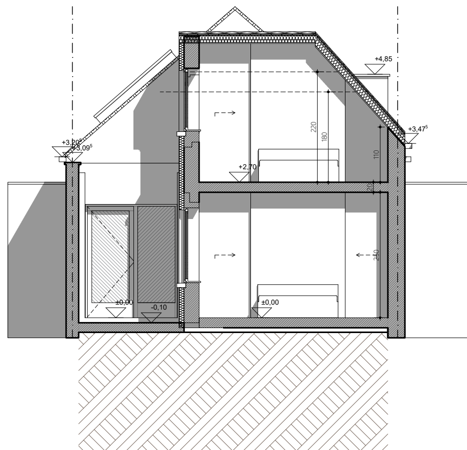
doorsnede BB - huidig Scheldestraat 72, 9040 Gent
