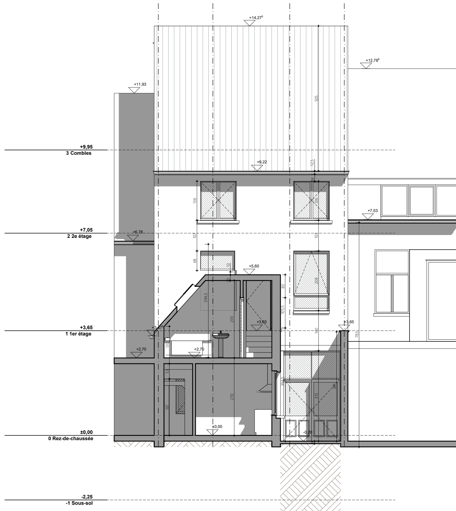
achtergevel + doorsnede CC - vergund Scheldestraat 72, 9040 Gent
