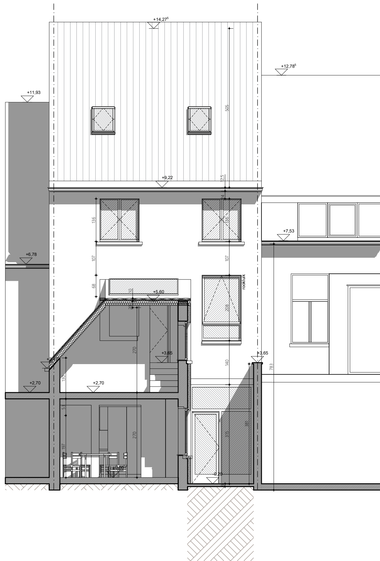
achtergevel + doorsnede CC - huidig Scheldestraat 72, 9040 Gent
