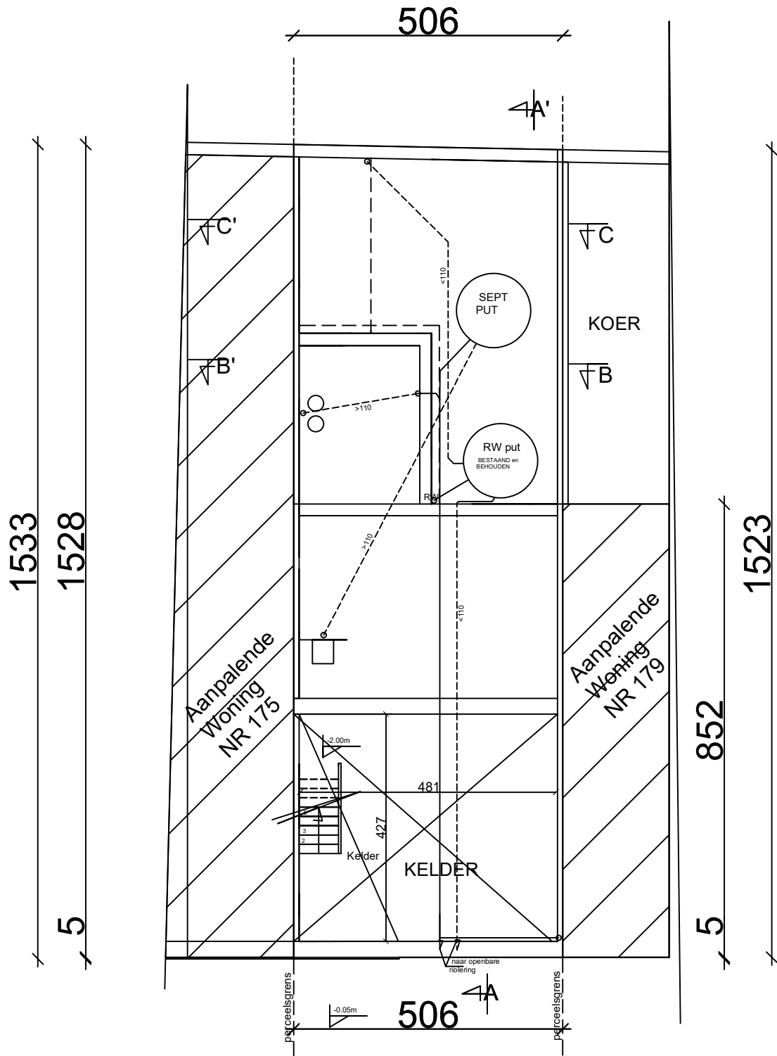
Kelder, funderings en rioleringsplan 1/100 Bestaande toestand
