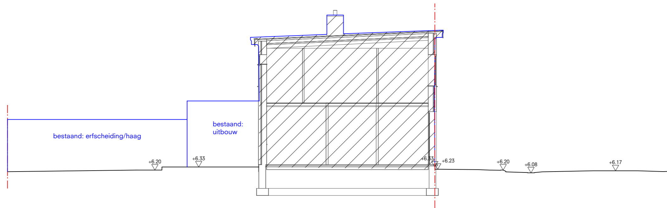
JG 2 linker- en rechtergevel bestaand aansluiting gabarit
