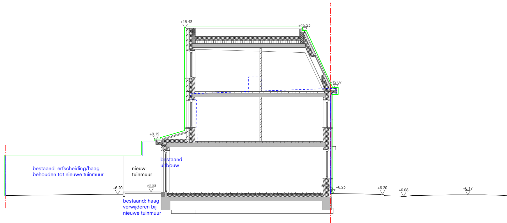
JG 2 linker- en rechtergevel aansluiting gabarit
