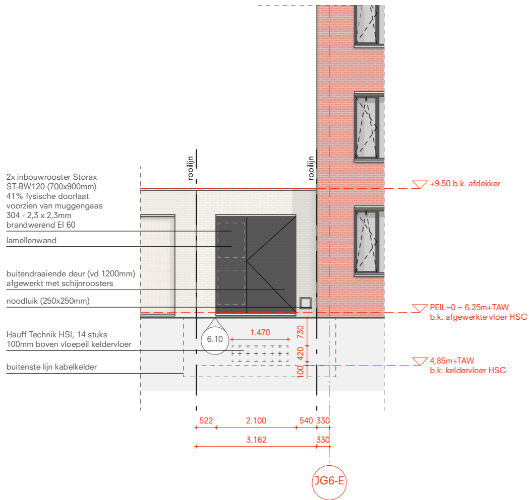
HSC Straatgevel
