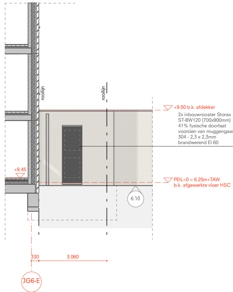
HSC Tuingevel
