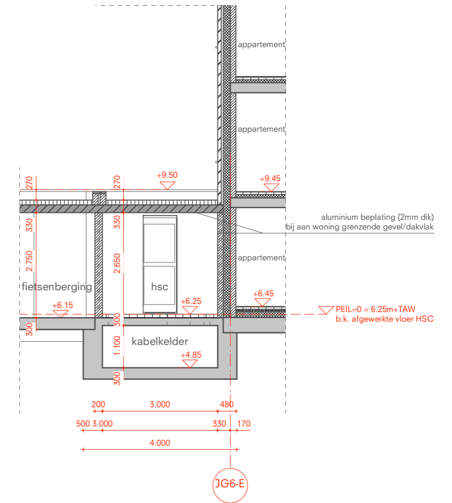
HSC Doorsnede
