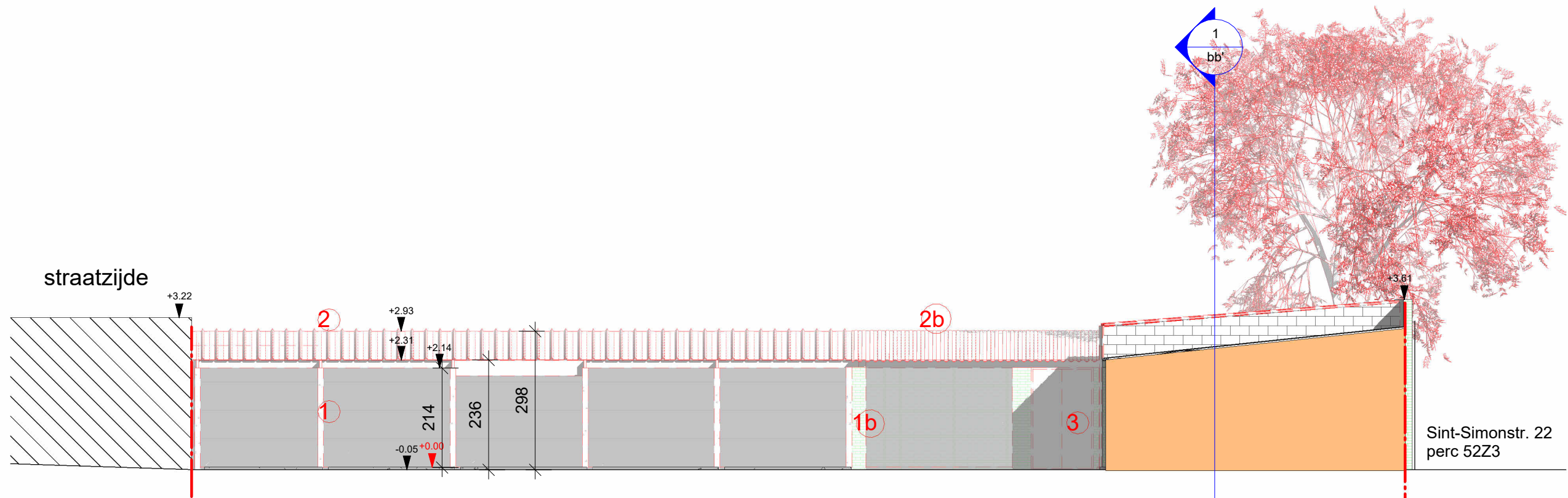
1 BA_garageboxen_G_V_2_rechteregevel 1 : 100
