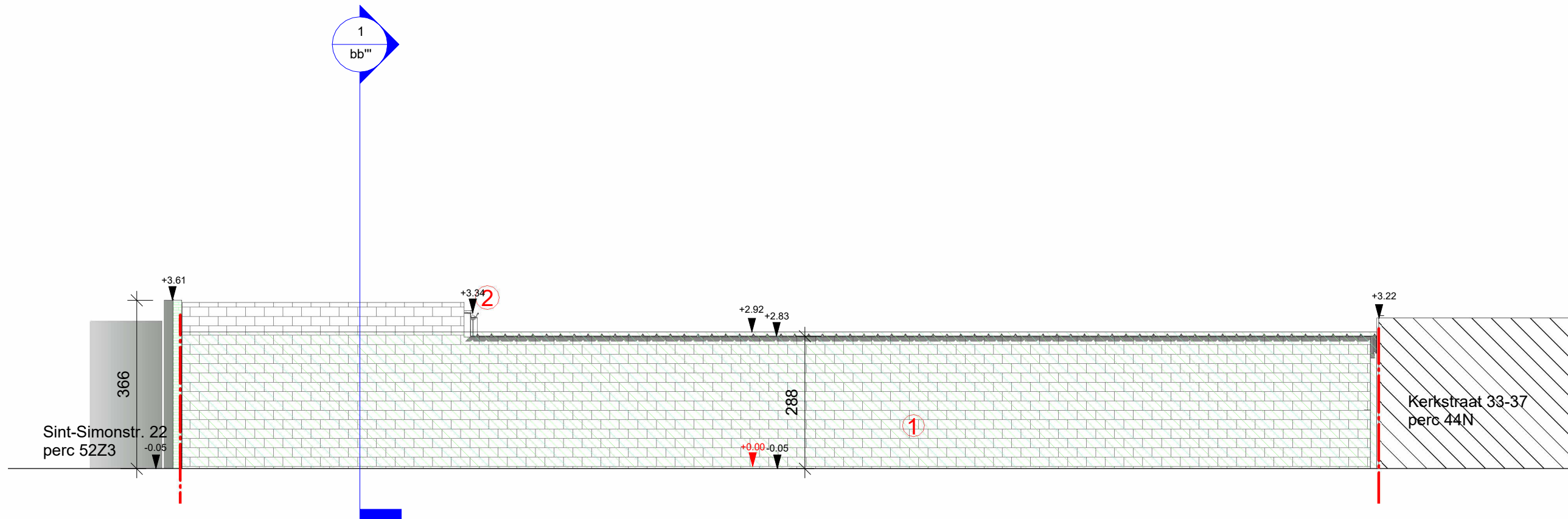
1 BA_garageboxen_G_N_4_linkergevel 1 : 100
