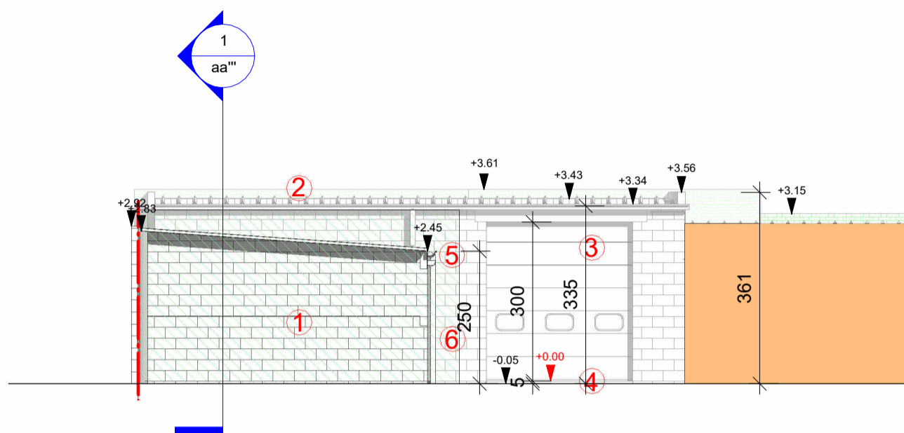
1 BA_garageboxen_G_N_1_voorgevel 1 : 100
