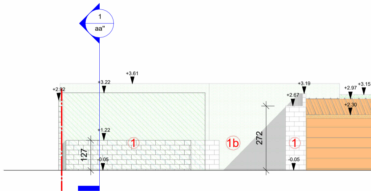
1 BA_garageboxen_G_B_1_voorgevel 1 : 100
