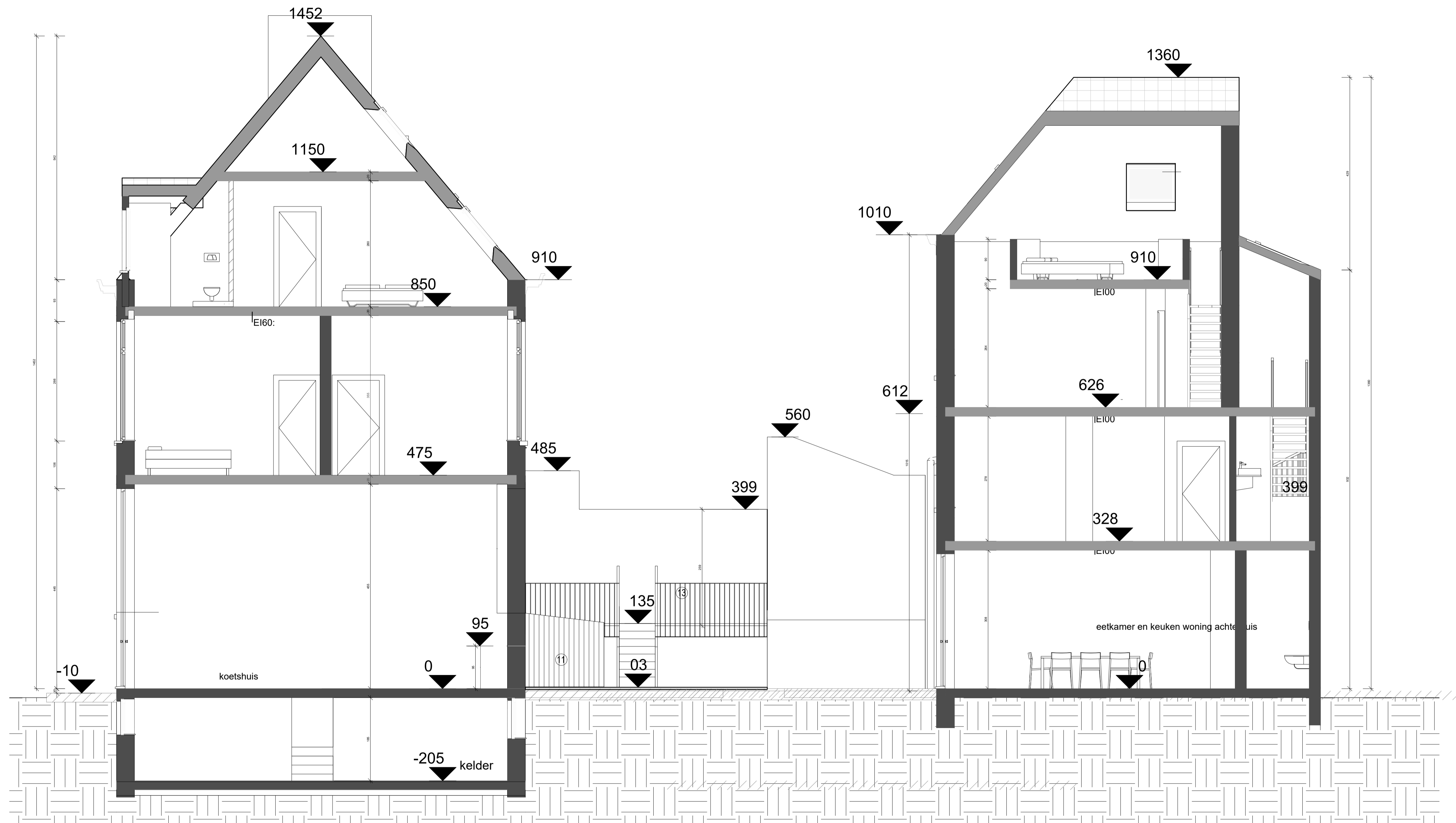
LANGSE SNEDE AA nieuwe toestand schaal: 1/100
