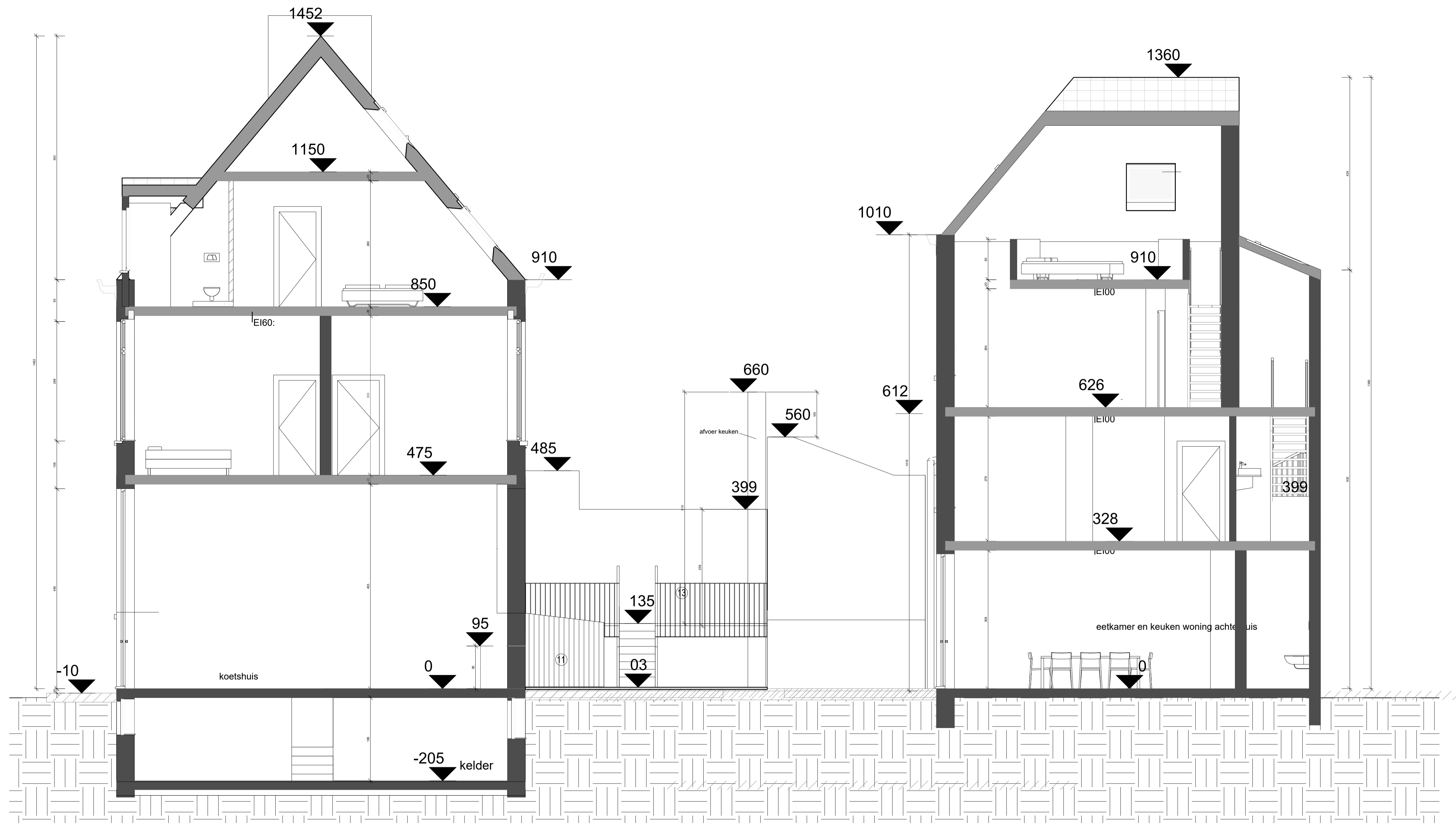
LANGSE SNEDE AA nieuwe toestand: update schaal: 1/100
