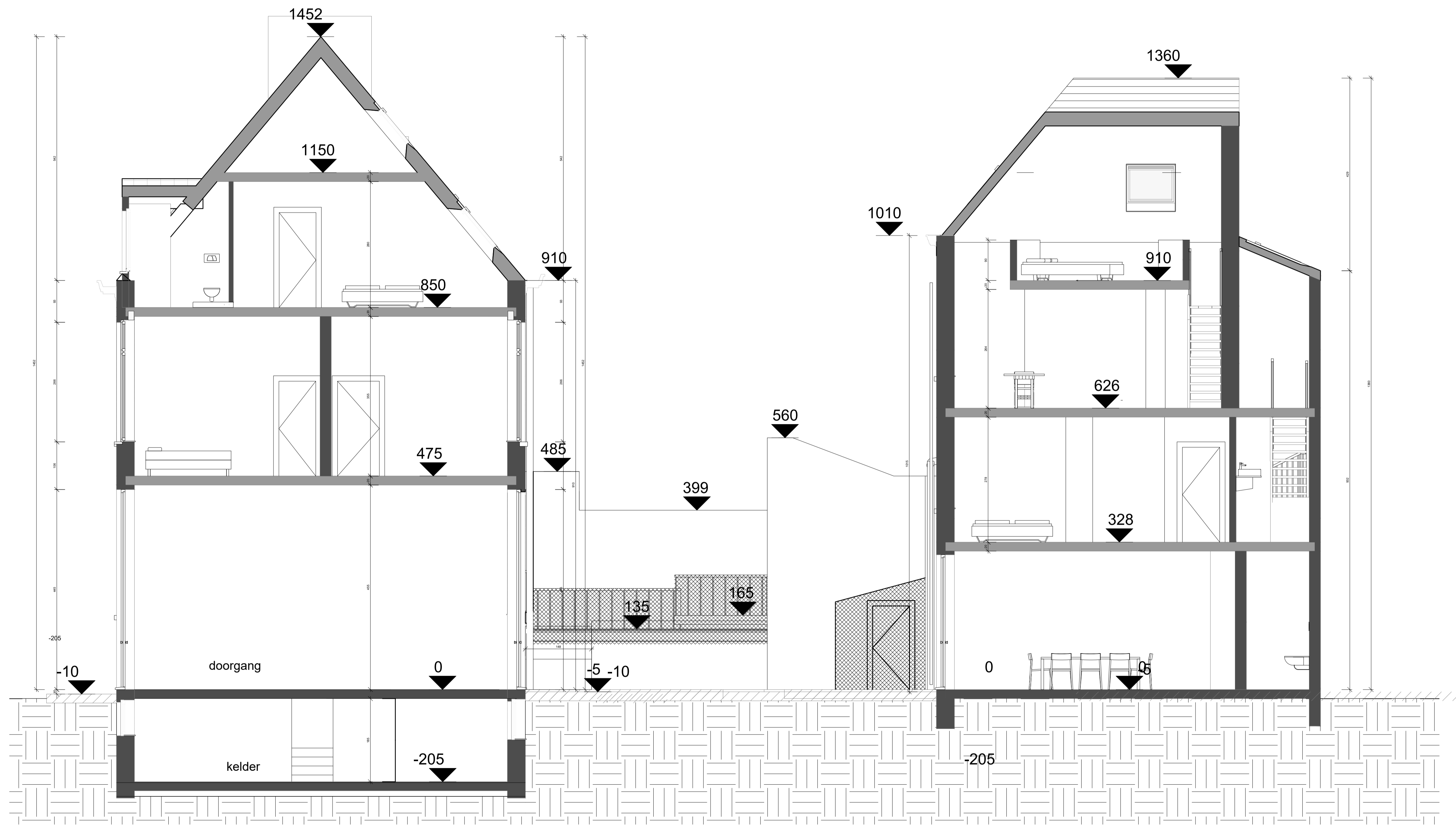
LANGSE SNEDE AA bestaande toestand schaal: 1/100
