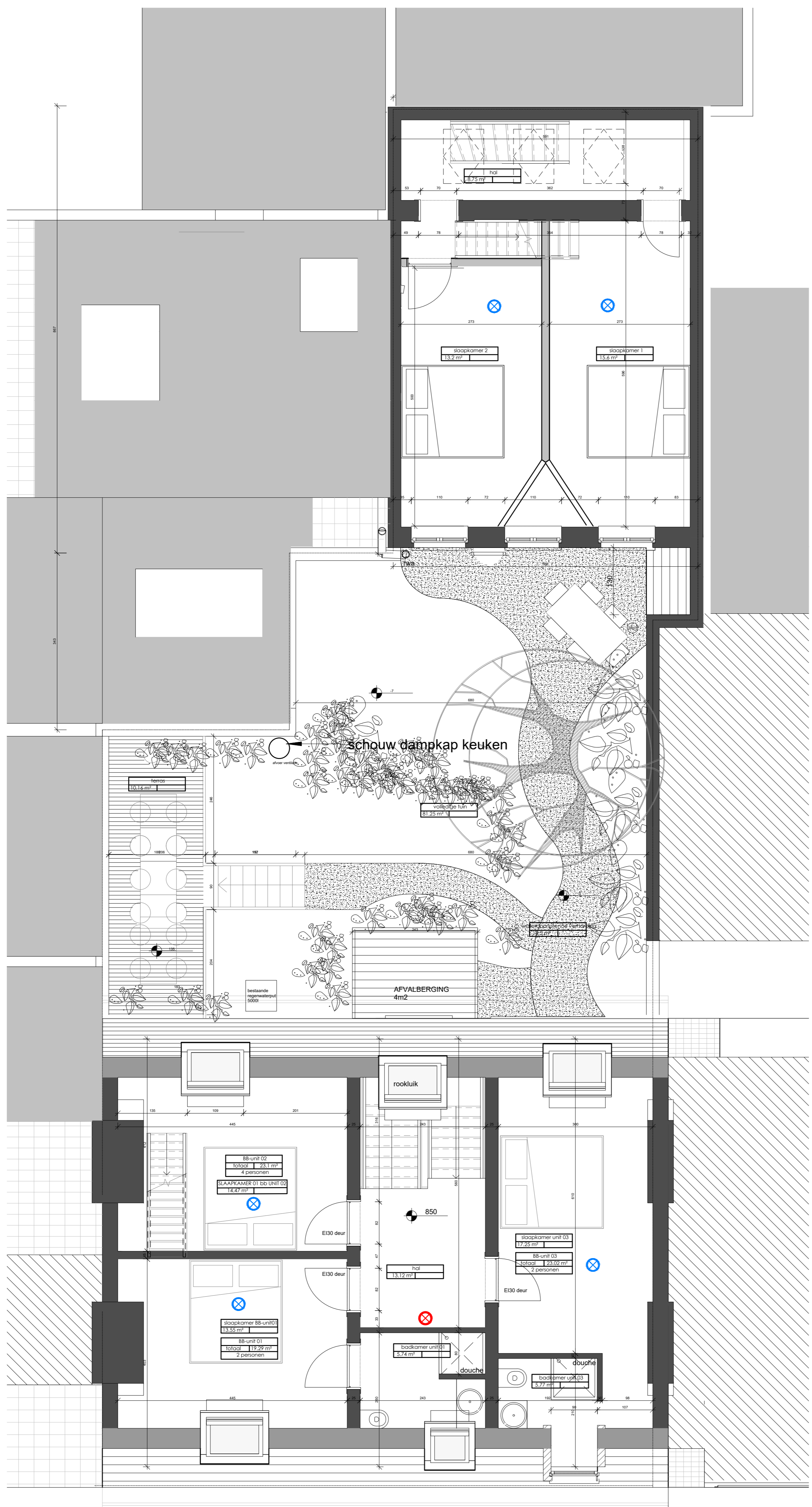
GRONDPLAN verdieping 2 nieuwe toestand schaal: 1/100
