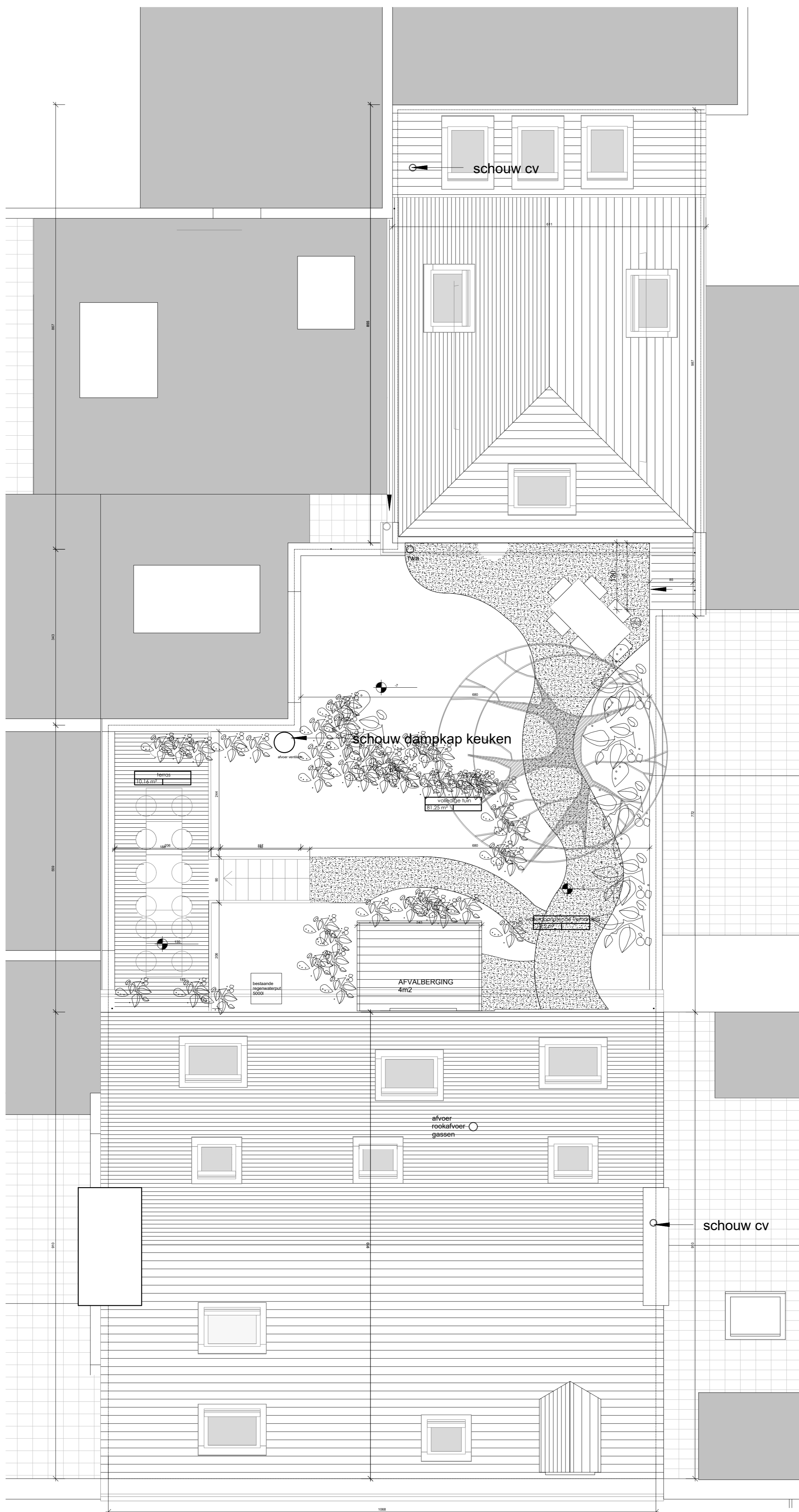
GRONDPLAN DAK nieuwe toestand schaal: 1/100
