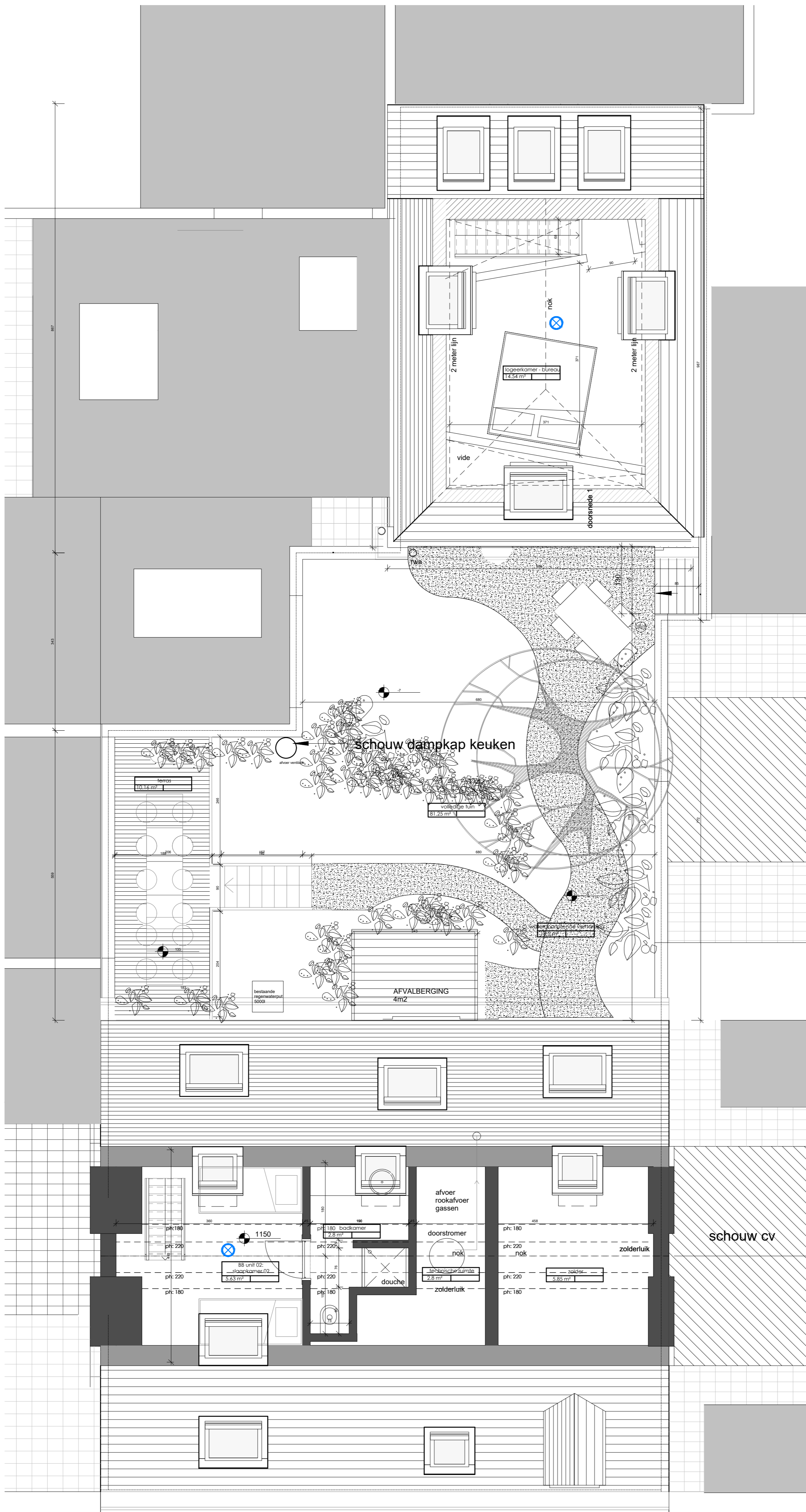
GRONDPLAN verdieping 3 nieuwe toestand schaal: 1/100
