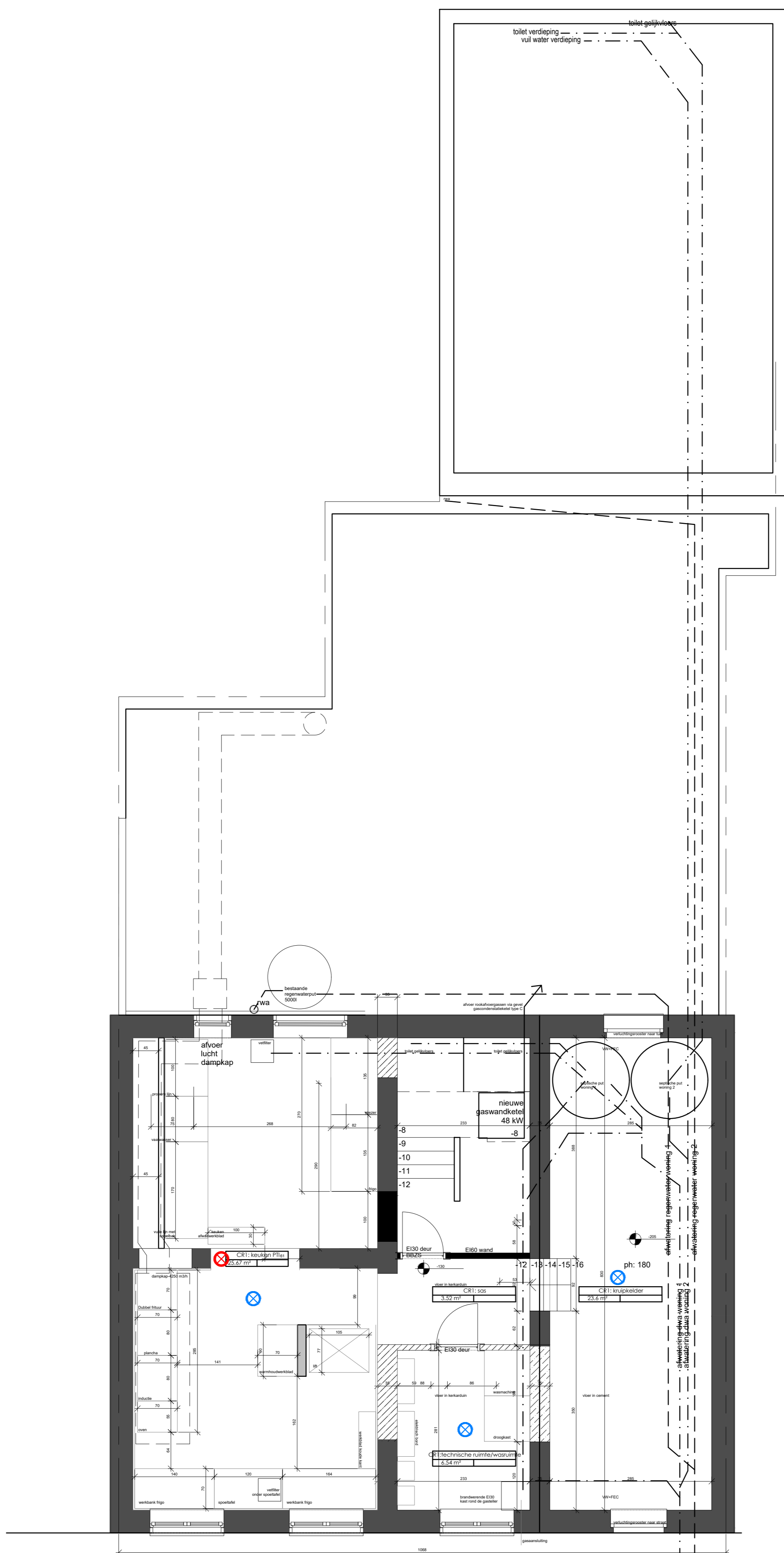
GRONDPLAN kelder en riolering nieuwe toestand: update schaal: 1/100
